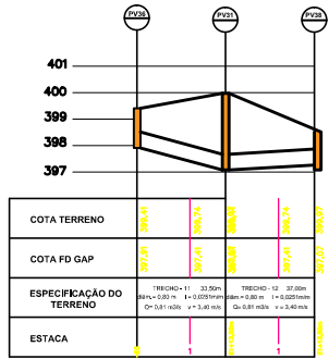
SUB-BACIA " g - 2 " PERFIL LONGITUDINAL DA GAP TRECHO - 11 E 12
