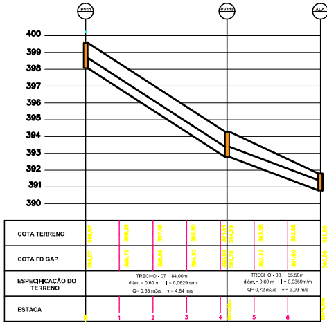
SUB-BACIA" D " PERFIL LONGITUDINAL DA GAP TRECHOS - 07 e 08
