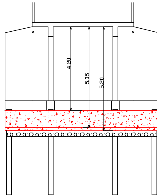
ELEVAÇÃO TRANSVERSAL ESC. 1:100
