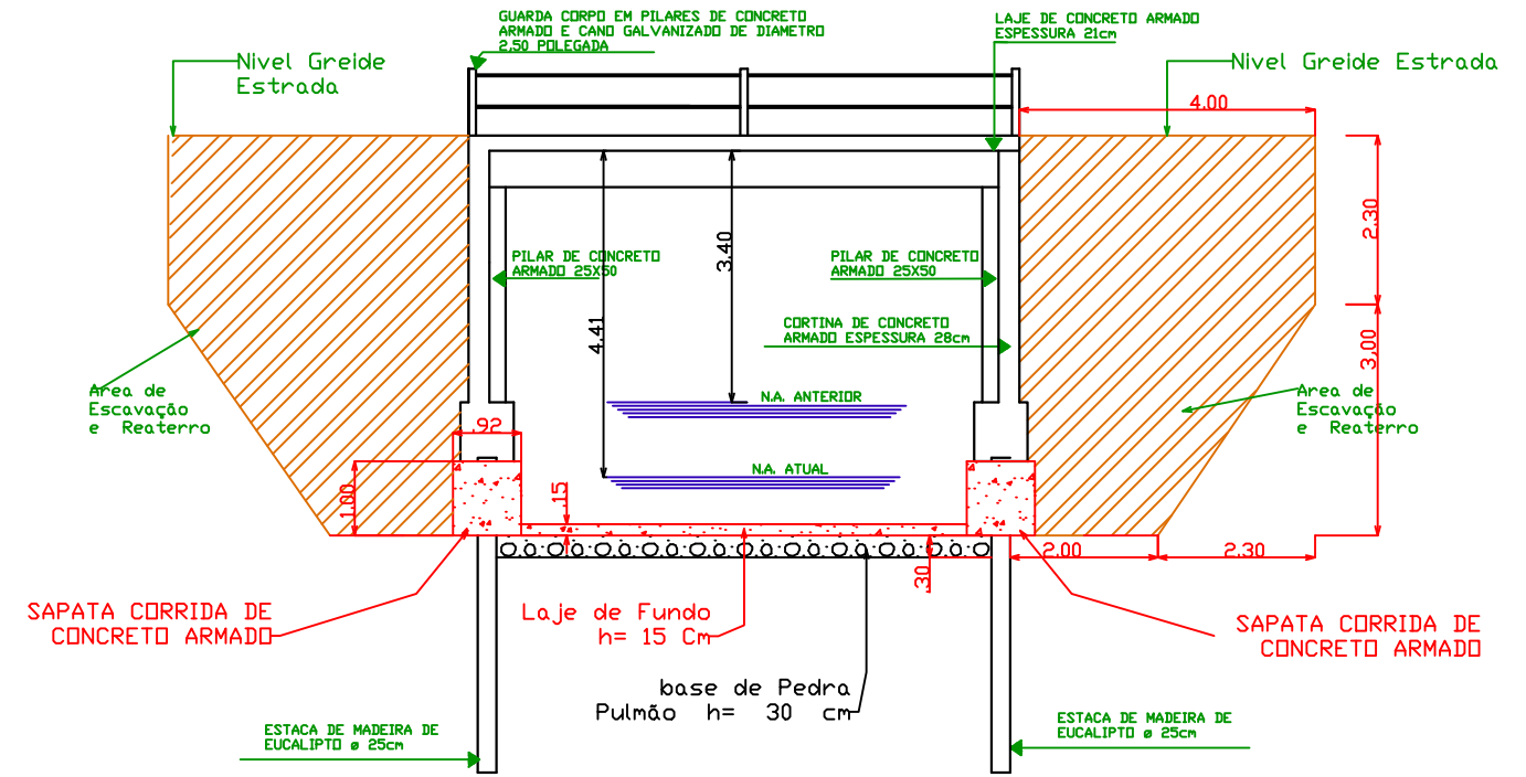
CORTE LOGITUDINAL ESC. 1:100
