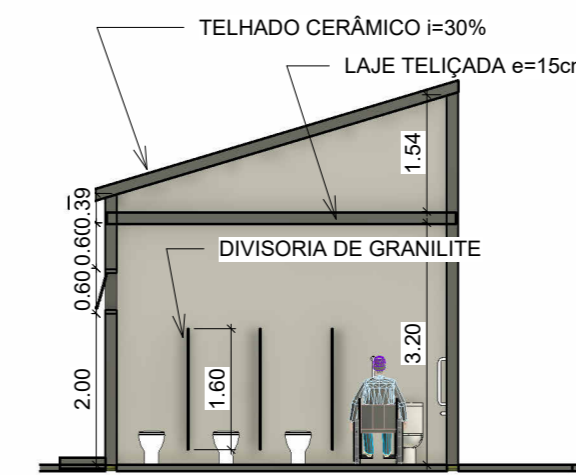
3 Corte 2 1 : 100
