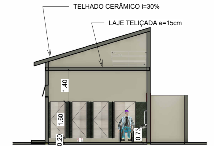
6 Corte 5 1 : 100
