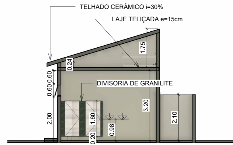
2 Corte 1 1 : 100
