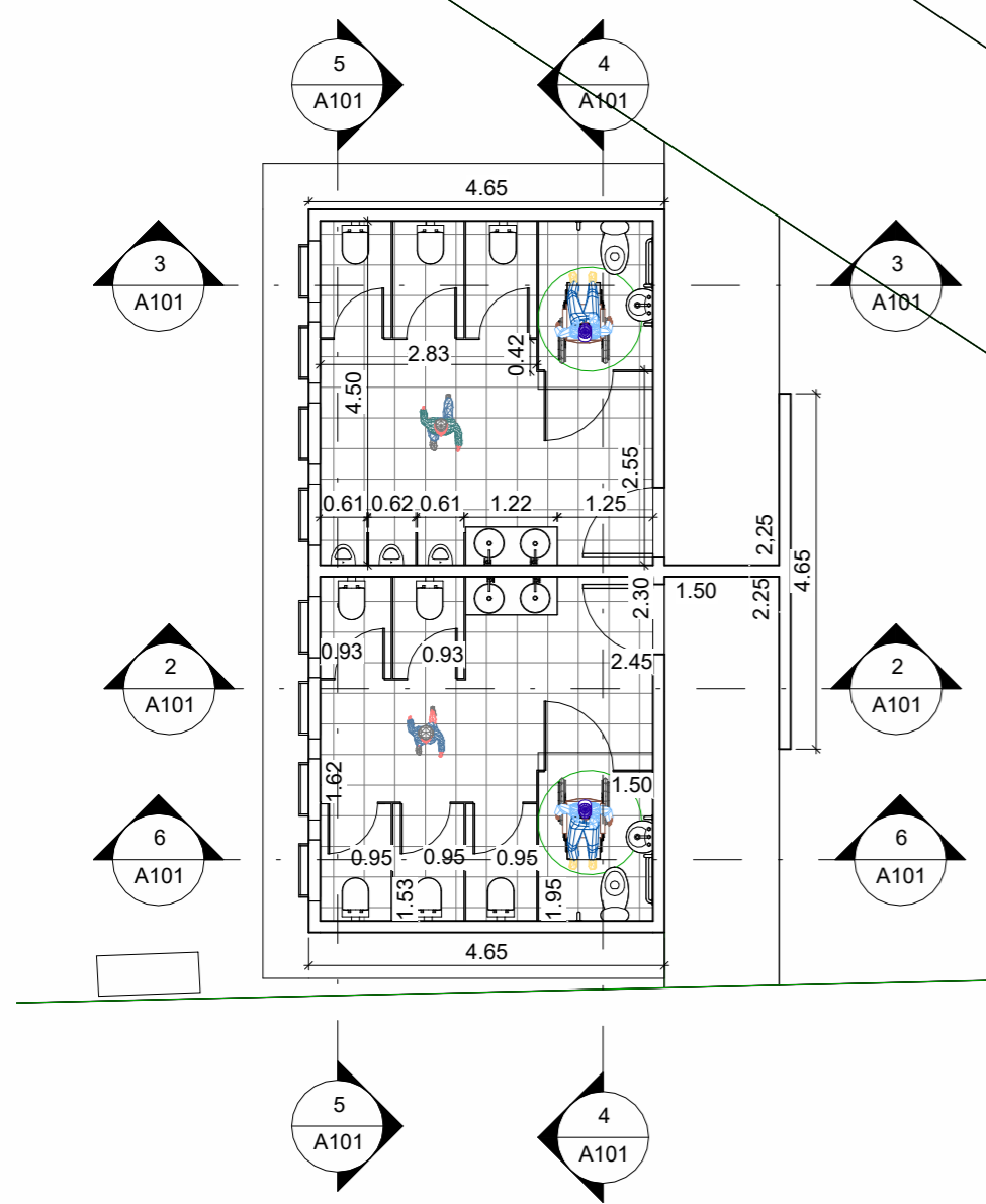
1 Planta Baixa 1 : 100
